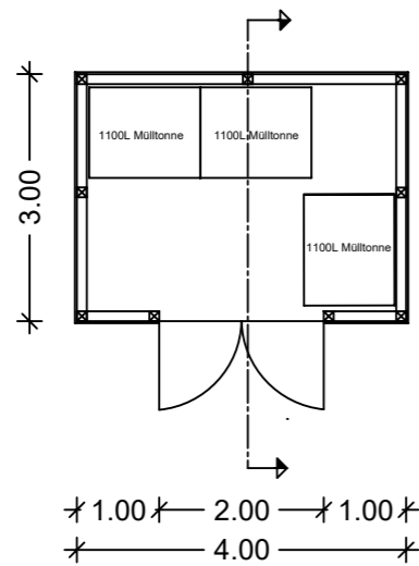
Grundriss
