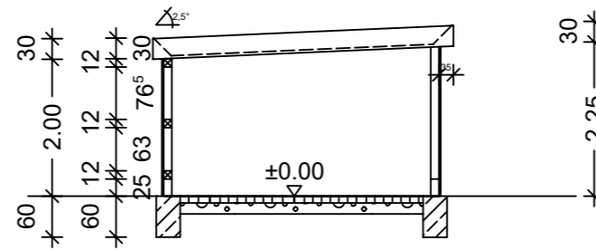
Schnitt A-A
